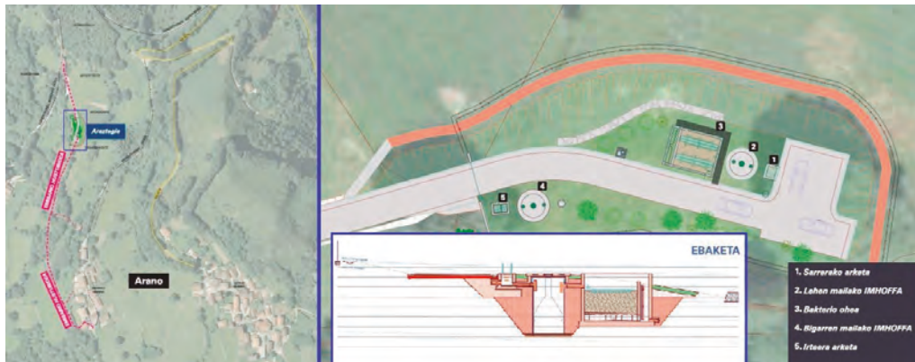
Araztegiaren planoak.
