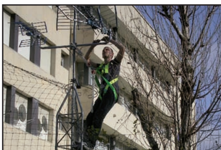
Telekomunikazioen elektronika
